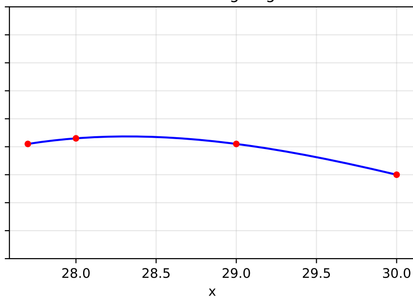
Curva 3: Lagrange
